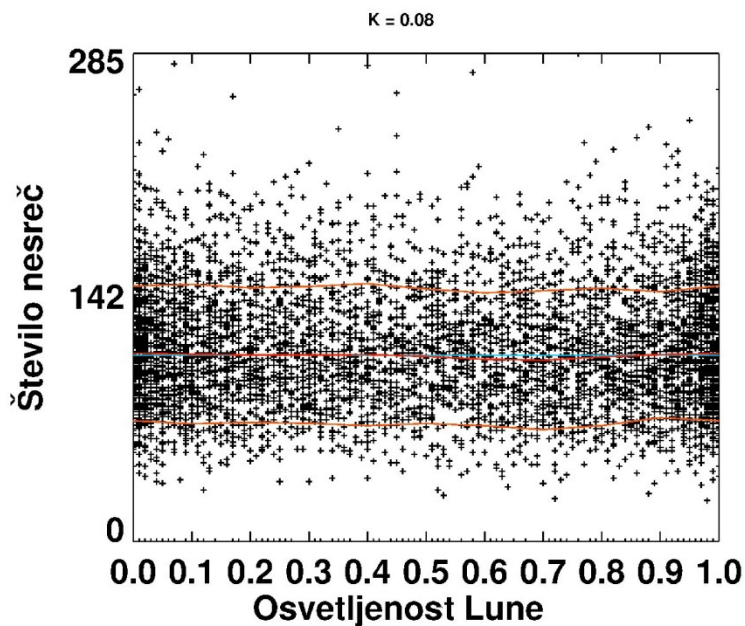
Slika 4. Število prometnih nesreč za vsak dan v obdobju od 1. 1. 1995 do 30. 6. 2010 v odvisnosti od navidezne osvetljenosti Lune.
